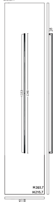
ANTA CESTELLO ESTRAIBILE PULL-OUT BASKET DRAWER DOOR
