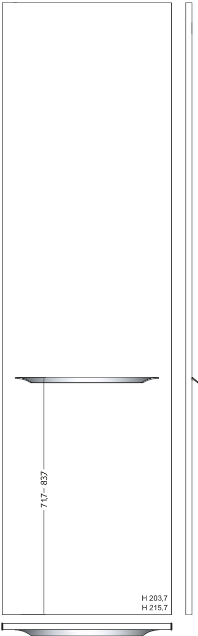
MANIGLIA FRONTALE PER ANTA COLONNA FRONT DOOR HANDLE FOR COLUMN
