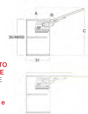
SCHEMA MONTAGGIO LIMITATORE PER RIBALTA H 36 FLAP DOOR LIMITER INSTALLATION DIAGRAM H 36
