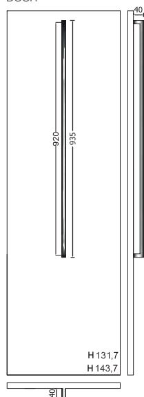
ANTA CESTELLO ESTRAIBILE PULL-OUT BASKET DRAWER DOOR
